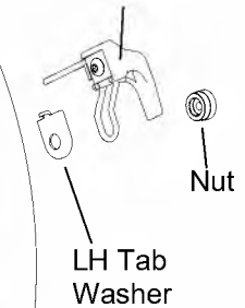
Hook Wire-Form
